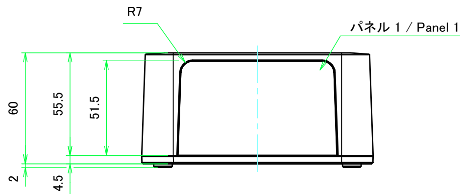
B-B ( 1 : 2 )
